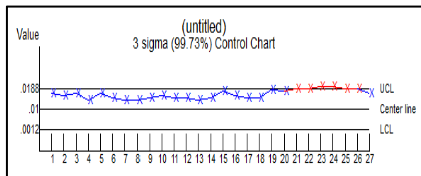
Gambar 12 Peta Kendali X (X-Chart) Dirty / Kadar Kotoran dalam Minyak (DIRT) Storage Tank nomor IV dan V Bulan Mei 2016
