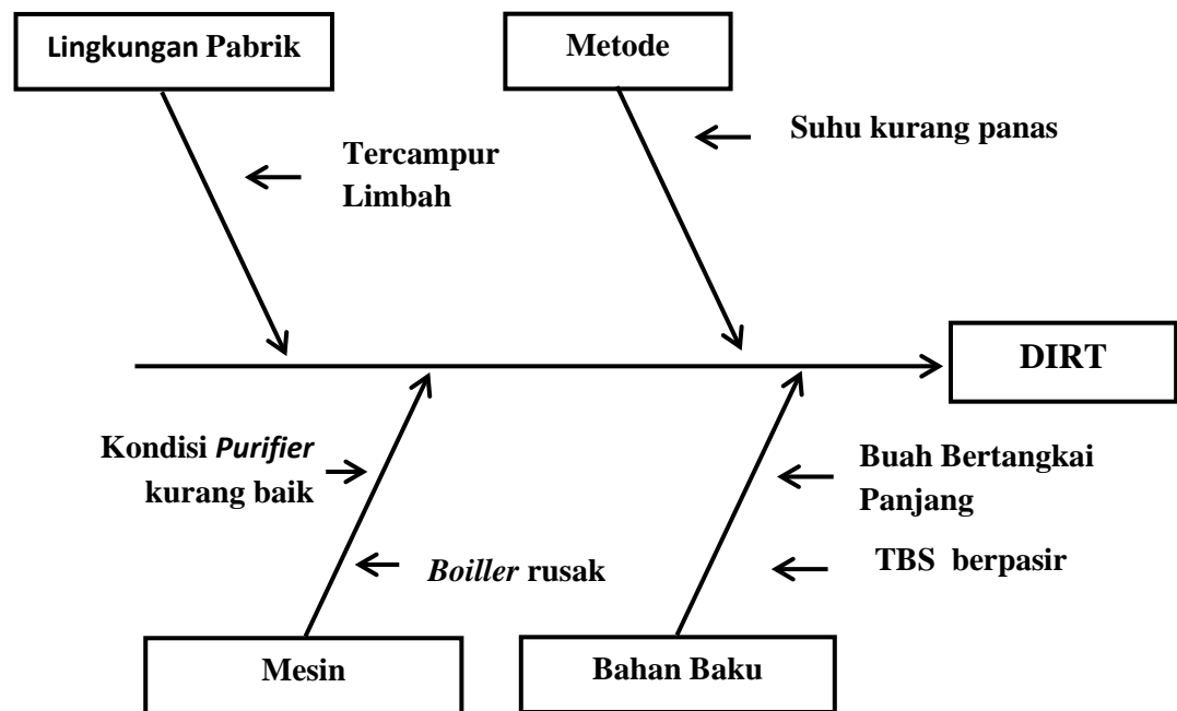
Gambar.9 Diagram Sebab Akibat Penyebab Tingginya Kadar Dirty / Kadar Kotoran dalam Minyak (DIRT) Oil Production Line I dan II Bulan Mei 2016
