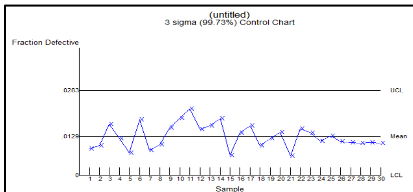
Gambar 1 Peta Kendali p (P-Chart) Penerimaan Tandan Buah Segar PT. Kalimantan Sanggar Pusaka Bulan Mei 2016
