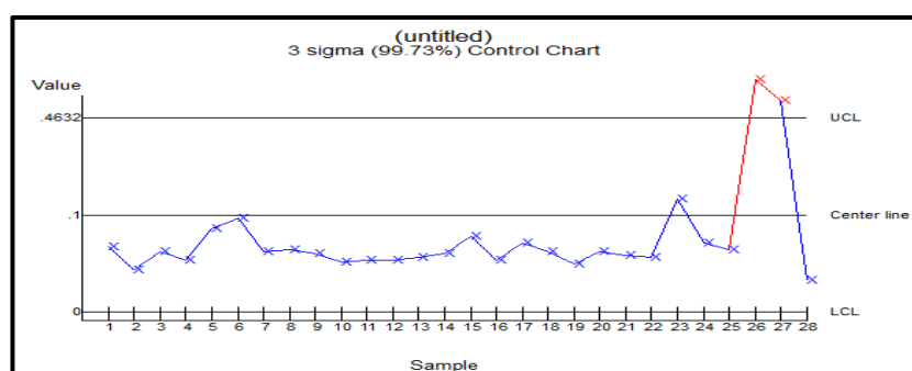
Gambar 5 Peta Kendali X ( X -Chart) Moisture / Kadar Air dalam Minyak (MOIST) Oil Production Line I dan II Bulan Mei 2016
