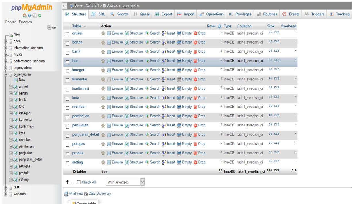
Gambar 4.2 Pembuatan Database menggunakan phpMyAdmin
