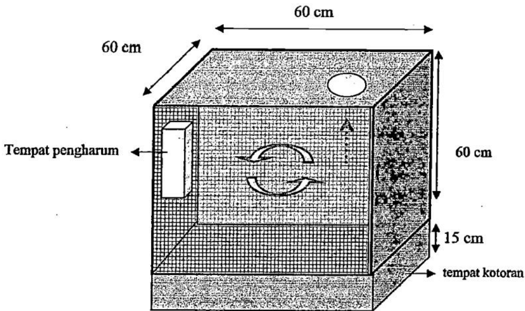
Gambar 3. Kandang perlakuan
