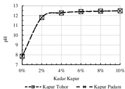
Gambar 1. Pengujian pH untuk menentukan ICL
