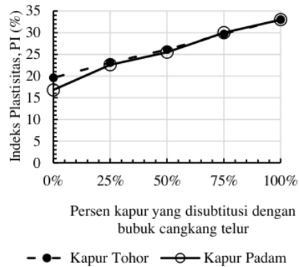
Gambar 5. Perbandingan jenis kapur terhadap plastisitas
