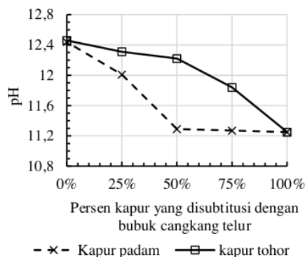
Gambar 2. Pengukuran pH campuran tanah-kapur-bubuk cangkang telur
