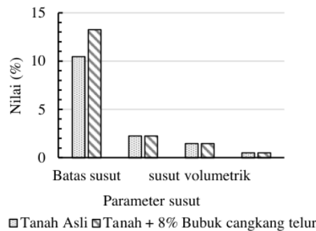
Gambar 7. Perbandingan parameter susut tanah asli dan tanah dengan stabilisasi bubuk cangkang telur
