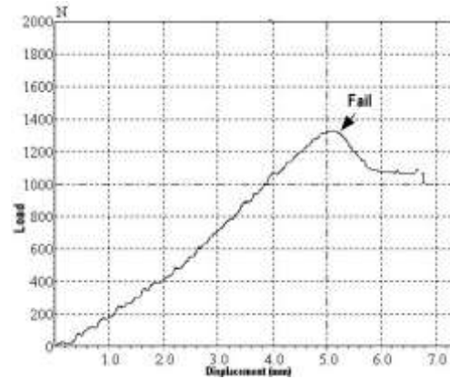
Gambar 7. Grafik beban-perpendekan
