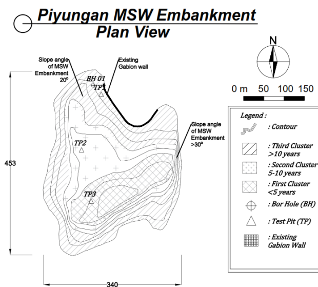
Fig. 2. Piyungan MSW embankment
