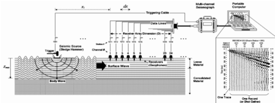
Gambar 1. Konfigurasi penentuan letak sensor dalam MASW
