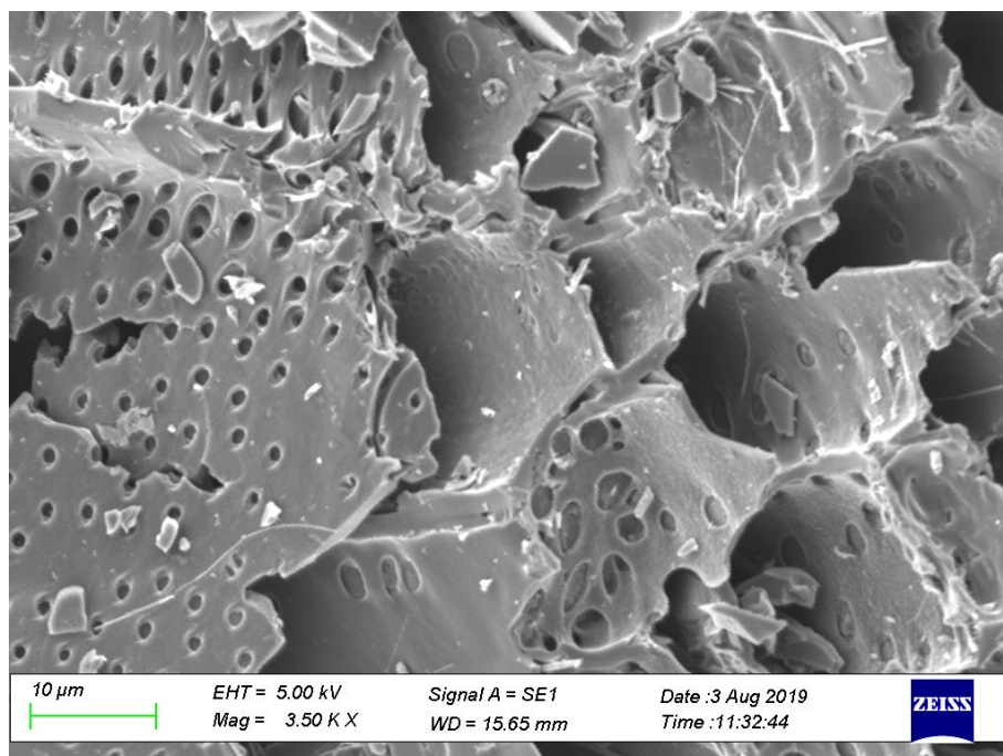
Pembesaran 3500 kali
