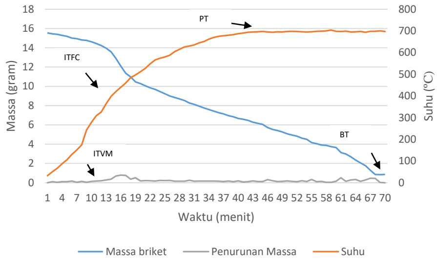
Grafik 50% kayu jati tekanan 750 Psi
