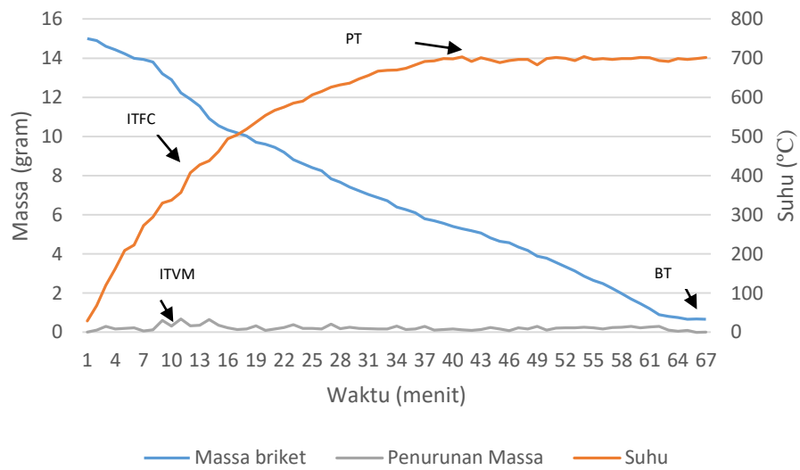
60% kayu jati tekanan 250 Psi
