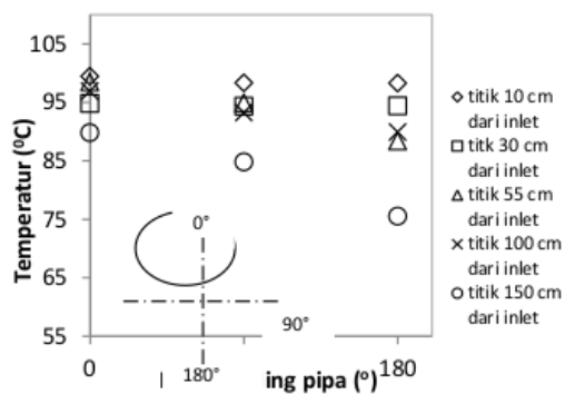
Gambar 2. Tipikal profil temperatur terhadap posisi keliling pipa ( \dot{m}_{s1} = 6,5 \times 10^{-3} \text{ kg/s} , \dot{m}_{c0} = 4,23 \times 10^{-1} \text{ kg/s} ).
