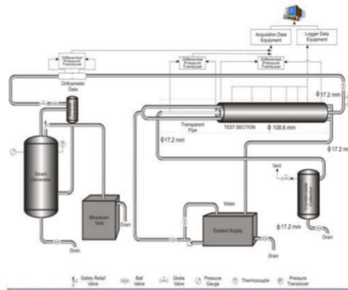
Gambar 1. Skema instalasi alat uji
