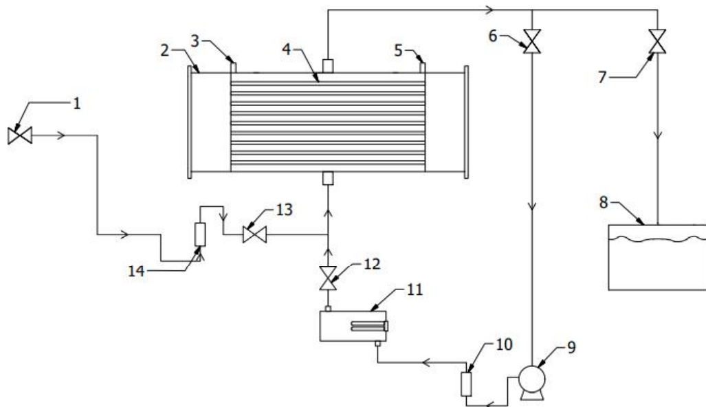
Gambar 3. 3 Skema aliran alat
