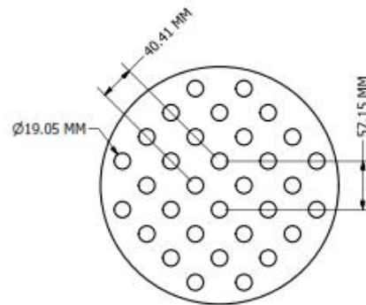
Gambar 3. 8 Susunan tube tembaga
