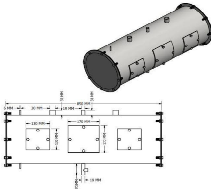
Gambar 3. 5 Tangki tampak 2 dimensi
