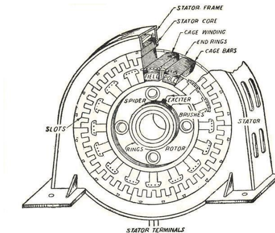
Gambar 2.2 Konstruksi Generator Sinkron (Ennopati, 2009)
