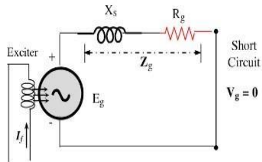
Gambar 2.13 Rangkaian Generator Pada Kondisi Hubung Singkat Satu Fasa
