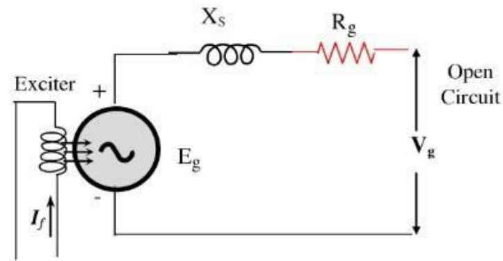
Gambar 2.11 Rangkaian Generator Sinkron Pada Kondisi Open Circuit (Muslim, 2008)
