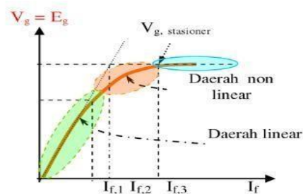
Gambar 2.12 Kurva V_g Terhadap I_f Pada Kondisi Open Circuit (Muslim, 2008)
