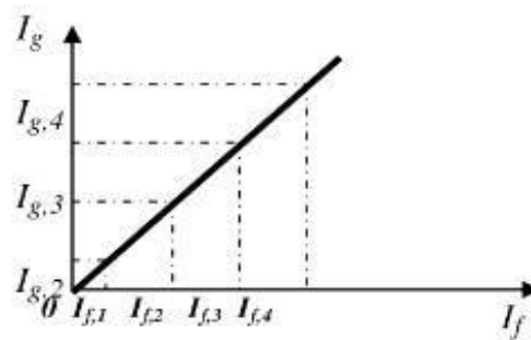
Gambar 2.15 Karakteristik Pada Kondisi Hubung Singkat
