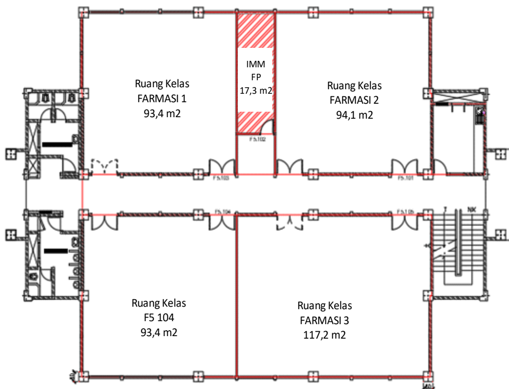
Gambar Denah Ruang F5 Lantai Satu
