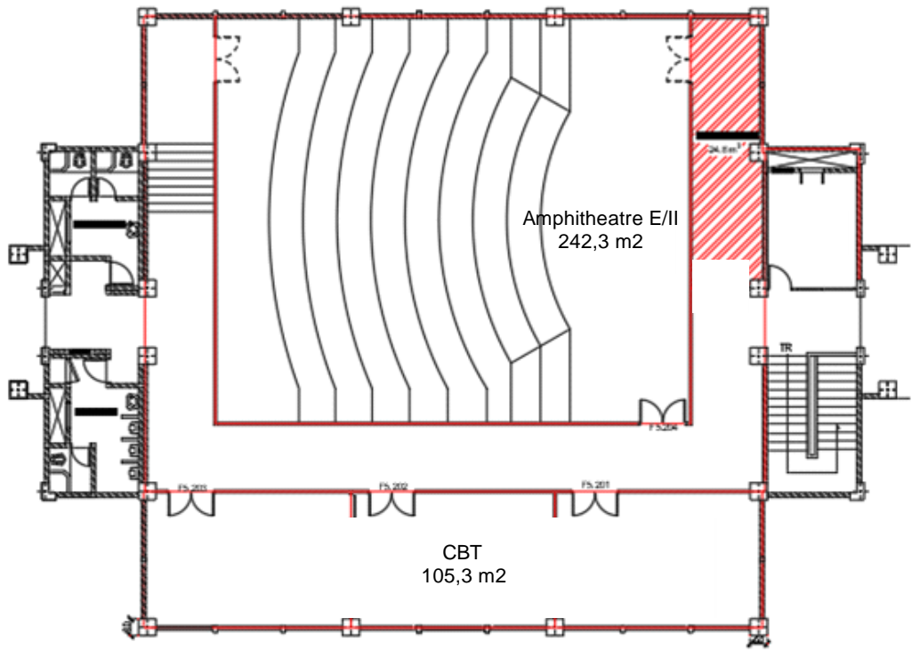
Gambar Denah Ruang F5 Lantai Dua
