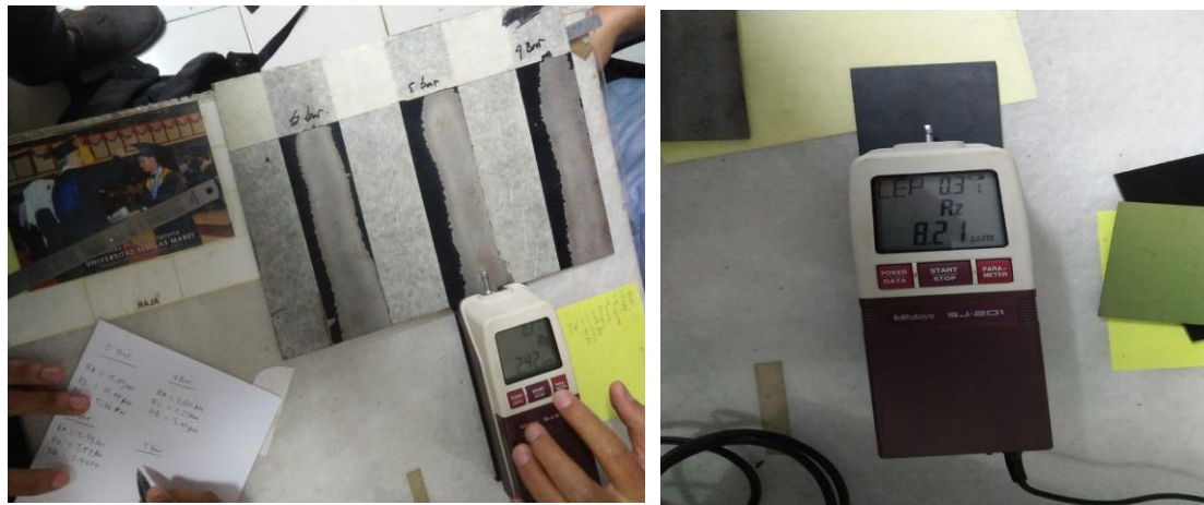
Gambar 1.5 Pengujian Kekasaran dengan Alat Surface Roughness Mitutoyo
