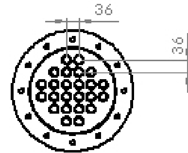
SECTION D-D SCALE 1 : 10
