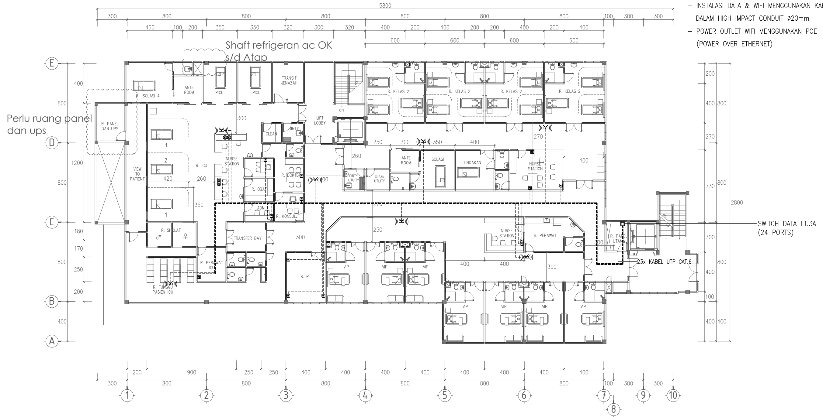
RENCANA DATA & WIFI (GEDUNG A) LANTAI 3 SKALA 1:200
