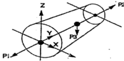
Gambar 3.30 Titik koneksi pada sebuah reducer
