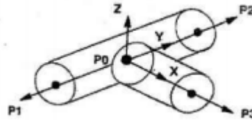
Gambar 3. 35 Titik-titik koneksi pada Tee .
