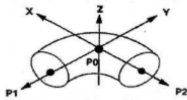
Gambar 3.32 Titik-titik koneksi pada Elbow atau Bend .
