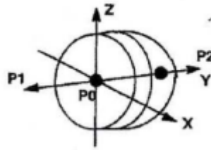
Gambar 3.34 Titik-titik koneksi pada Cap/Plug/Blind Flange .
