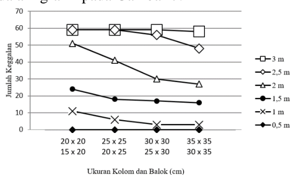
Gambar 7 Grafik kegagalan struktur bangunan rumah tinggal 2 lantai
