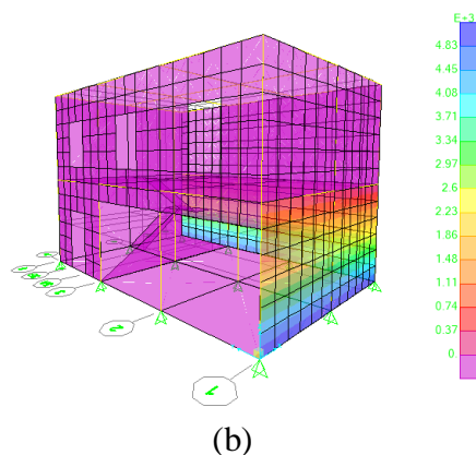
Gambar 3 Tekanan banjir lahar dingin 3 m pada bangunan rumah tinggal (a) 1 lantai, (b) 2 lantai.
