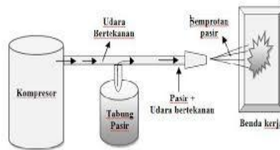
Gambar 2.1: Teknik sandblasting Sumber: (Setyarini dan Sulistyio 2011)
