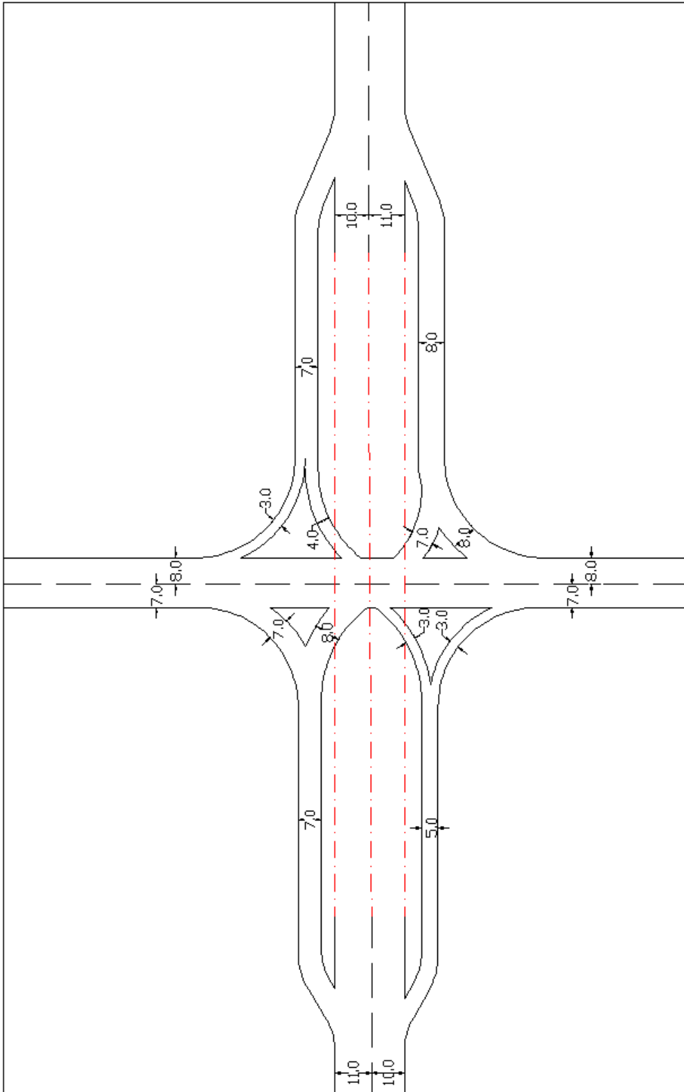
Lampiran 2. Desain geometrik Simpang SPUI Default
