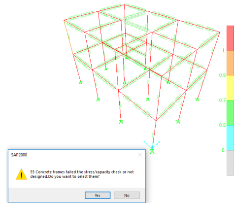
Gambar 10 Kolom 25 x 25 cm dan ketinggian banjir 2 m
