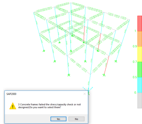
Gambar 20 Kolom 35 x 35 cm dan ketinggian banjir 1 m
