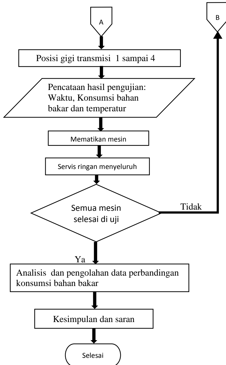
Gambar 3. 23 Diagram alir pengujian konsumsi bahan bakar (Lanjutan)
