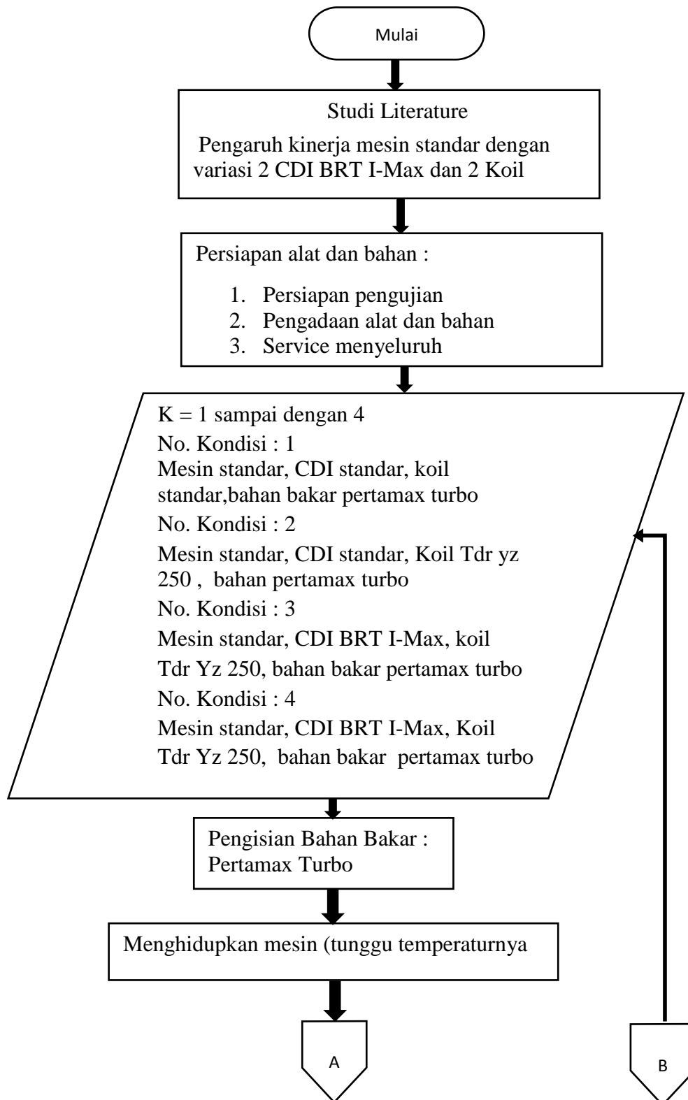
Gambar 3. 22 Diagram alir pengujian konsumsi bahan bakar
