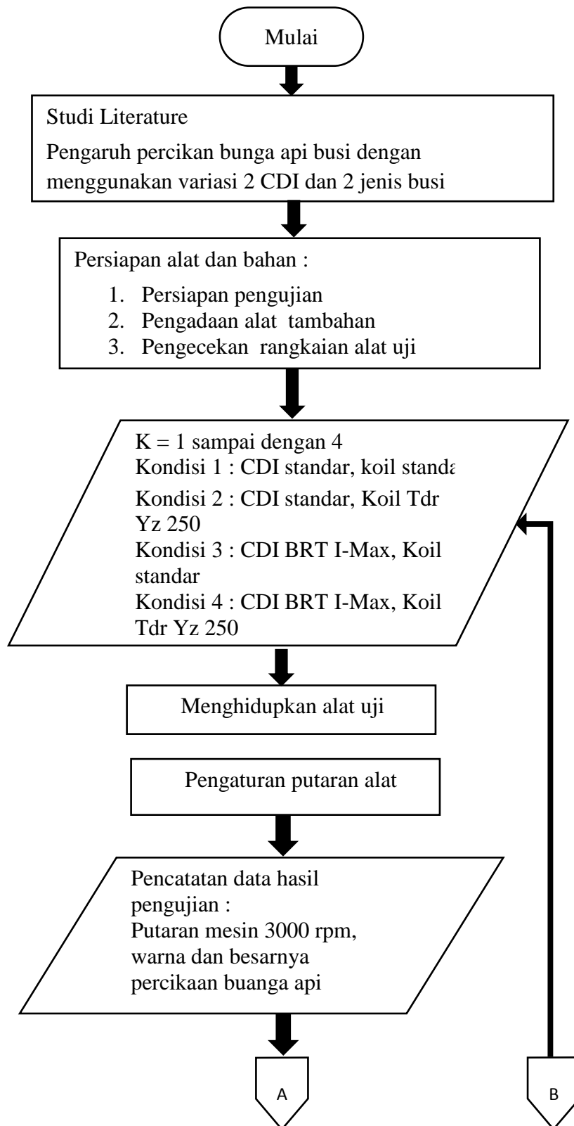
Gambar 3. 16 Diagram alir pengujian karakteristik bunga api
