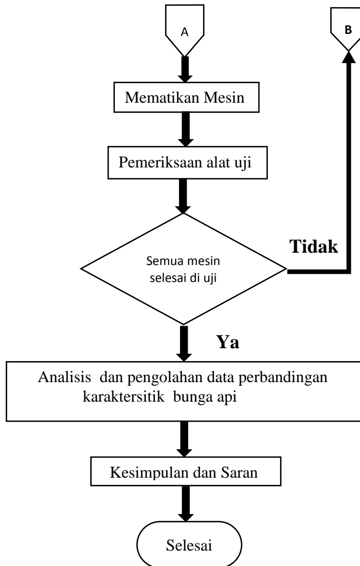
Gambar 3. 17 Diagram alir pengujian karakteristik bunga api (Lanjutan)
