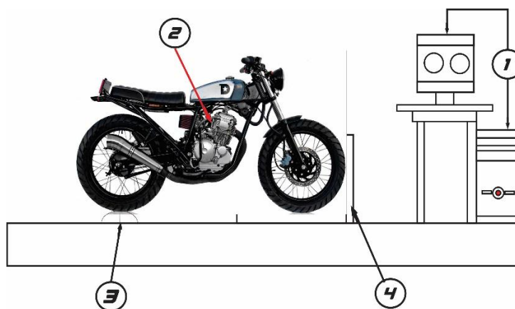
Gambar 3. 24 Alat Uji Dynamometer
