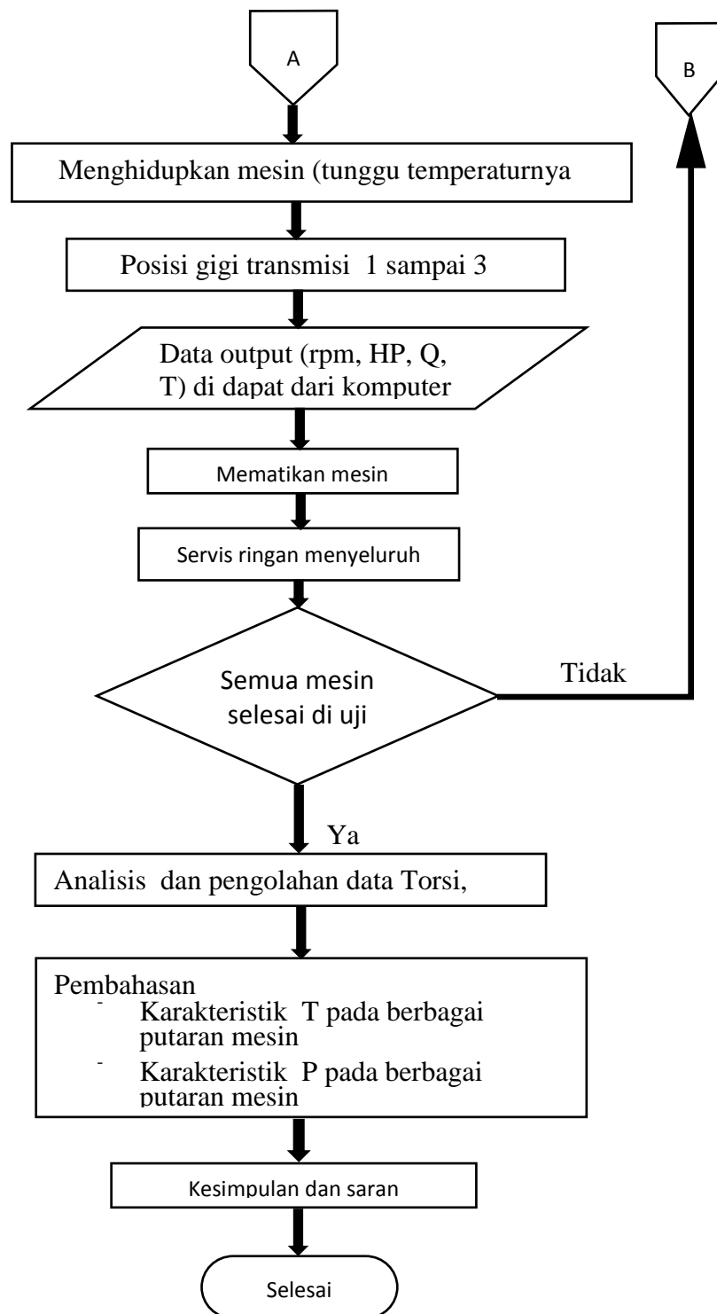
Gambar 3. 20 Diagram alir pengujian Torsi dan Daya (Lanjutan)
