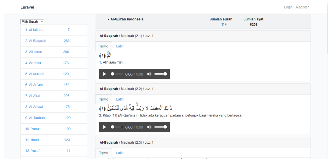
Gambar 4.7 Surah Lain
