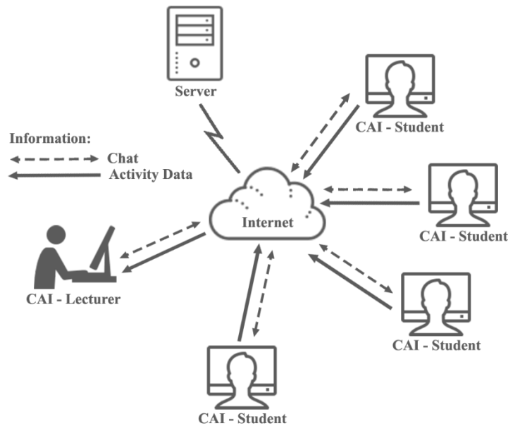
Gambar 1 Arsitektur CAI
