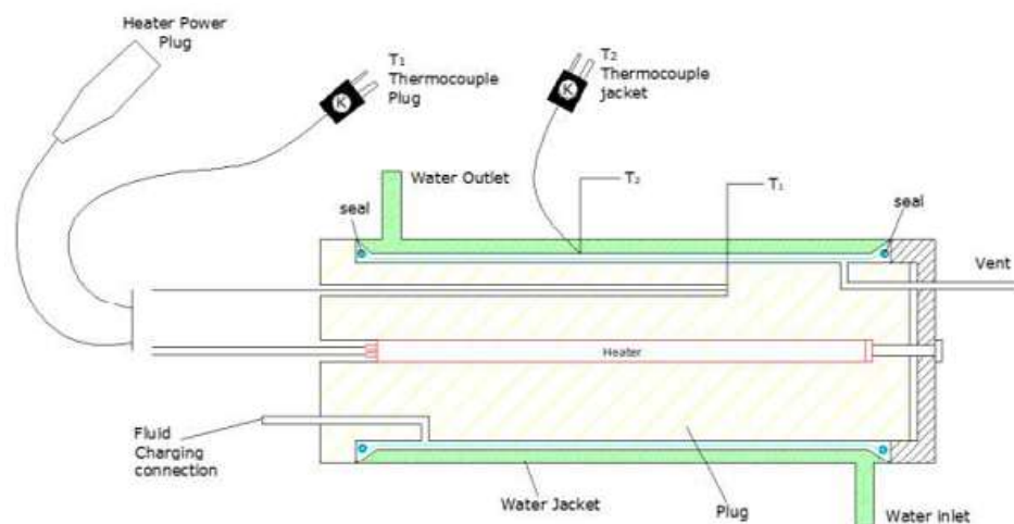
Gambar 2.2 Skema alat konduktivitas termal (Santosa dan Nurcahyadi, 2016)
