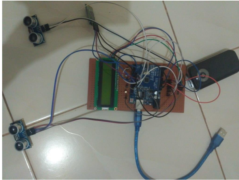
Gambar 1 Bentuk Keseluruhan Sistem
