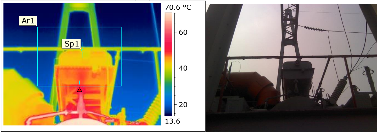
Picture 15. Captured at: Konsevator
