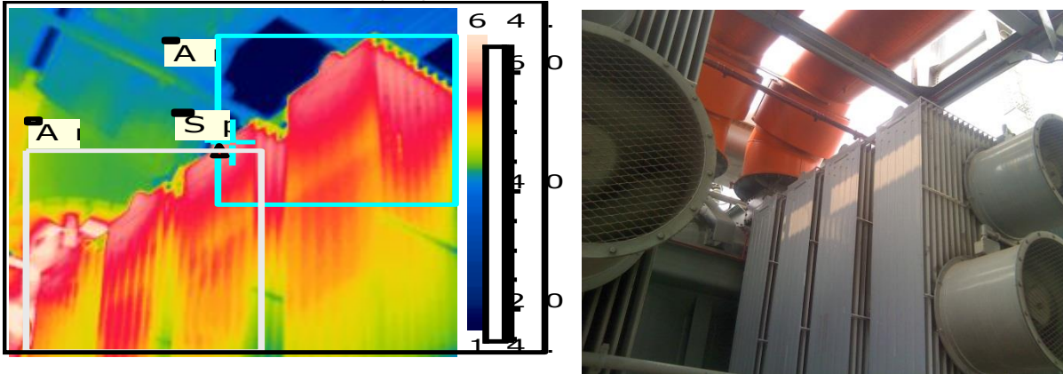
Picture 7. Captured at: fin pendingin sisi utara – barat (bagian dalam)
