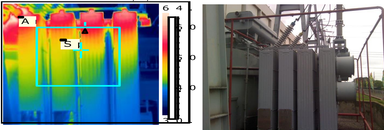
Picture 4. Captured at: fin pendingin sisi selatan – barat luar
