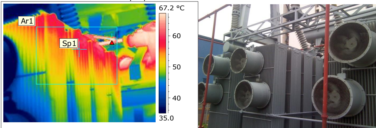
Picture 14. Captured at: fin pendingin sisi selatan – barat (bagian dalam)
