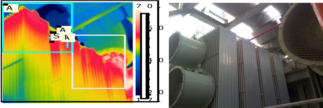
Picture 9. Captured at: fin pendingin sisi utara – timur (bagian dalam)
