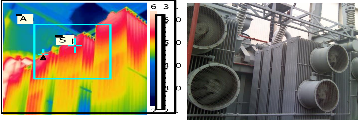
Picture 13. Captured at: fin pendingin sisi selatan – timur (bagian dalam)
