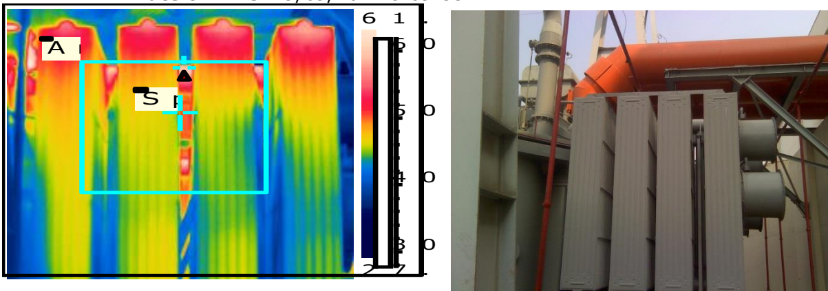
Picture 10. Captured at: fin pendingin sisi utara – timur (bagian luar)
