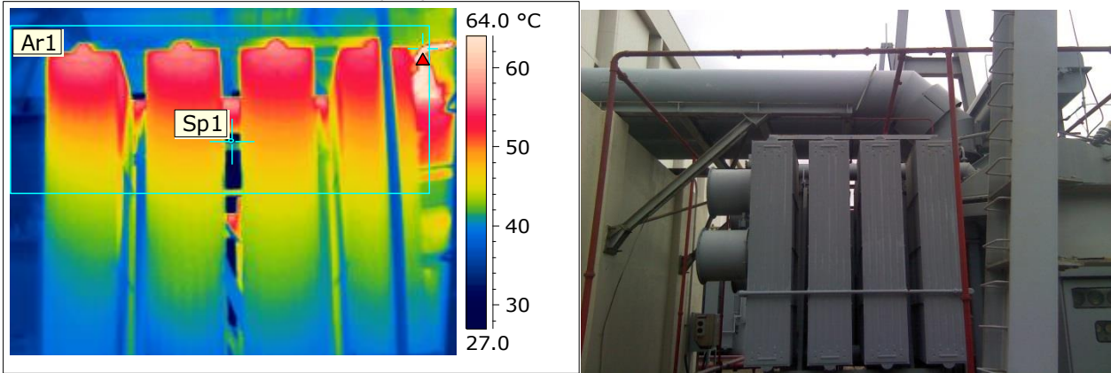
Picture 5. Captured at: fin pendingin sisi utara – barat (bagian luar)
