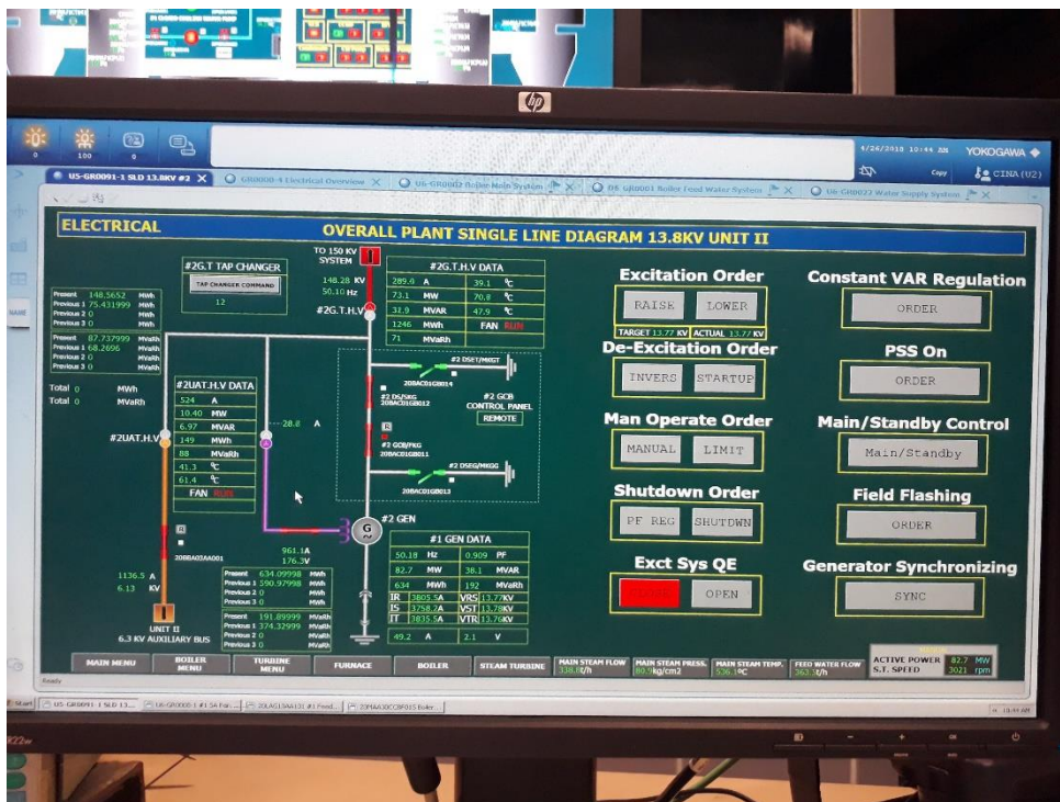
Gambar 5.4 Diagram Single Line Generator Pada Monitor
