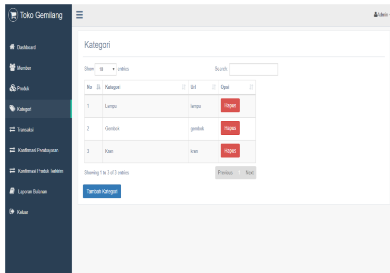
Gambar 4. 16 Halaman Kategori
