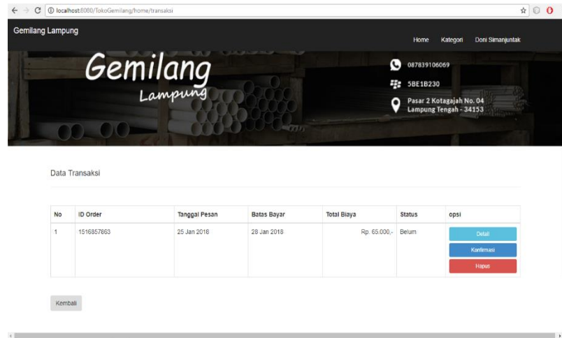
Gambar 4. 9 Halaman Transaksi
