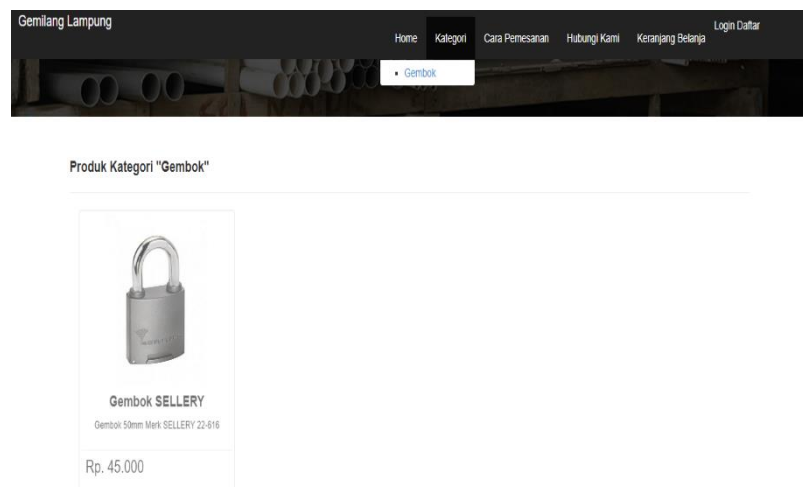
Gambar 4. 6 Halaman Kategori
