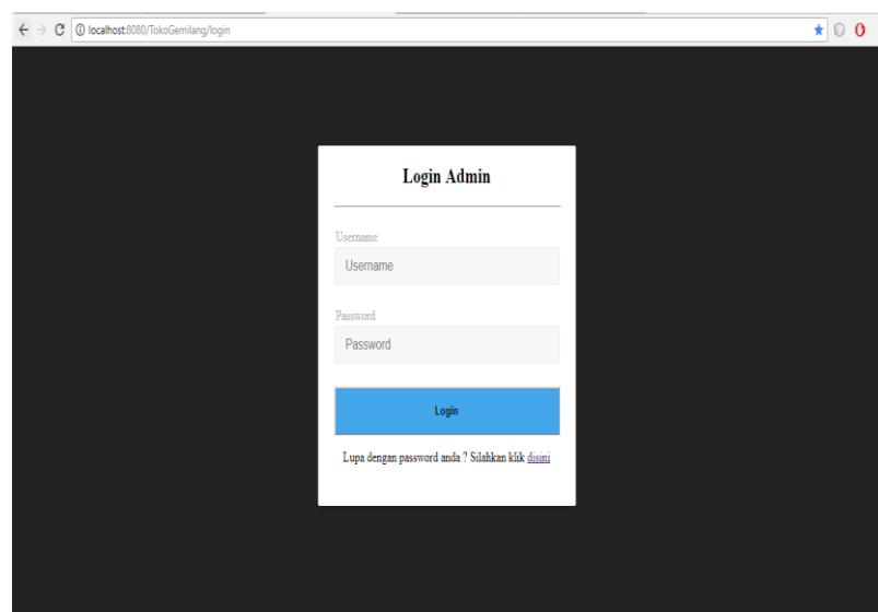
Gambar 4. 14 Halaman Login
