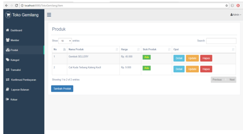
Gambar 4. 18 Halaman Produk
