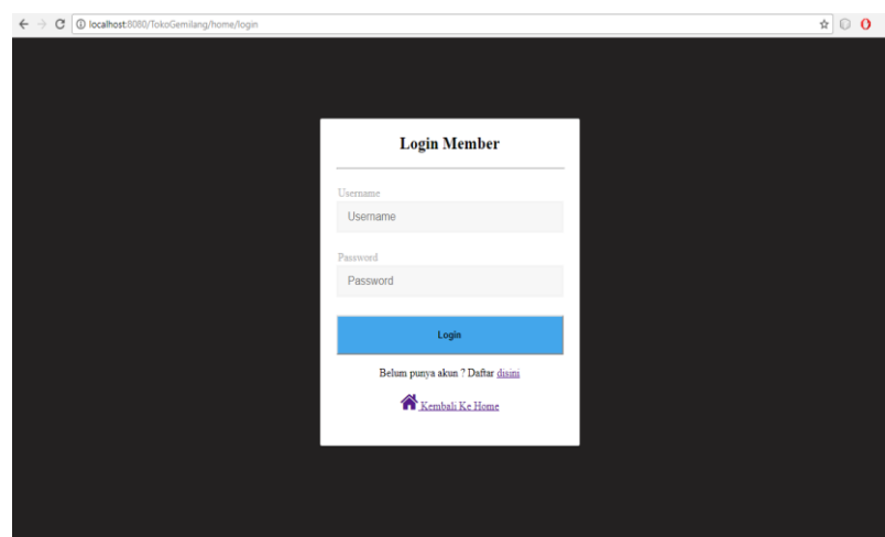
Gambar 4. 2 Halaman Login
