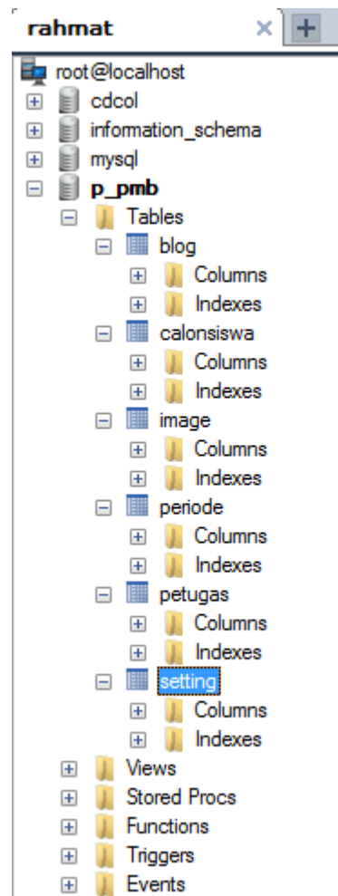
Gambar 4.1 Database Aplikasi
