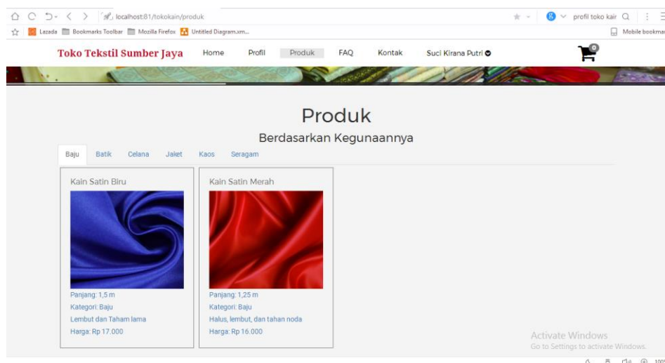
Gambar 4.13 Halaman Produk
