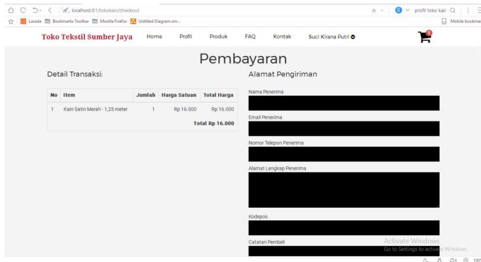
Gambar 4.16 Halaman Pembayaran
