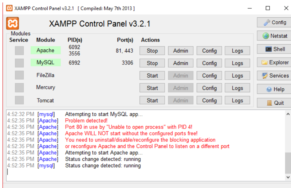
Gambar 4.1 Running Apache dan MySql
