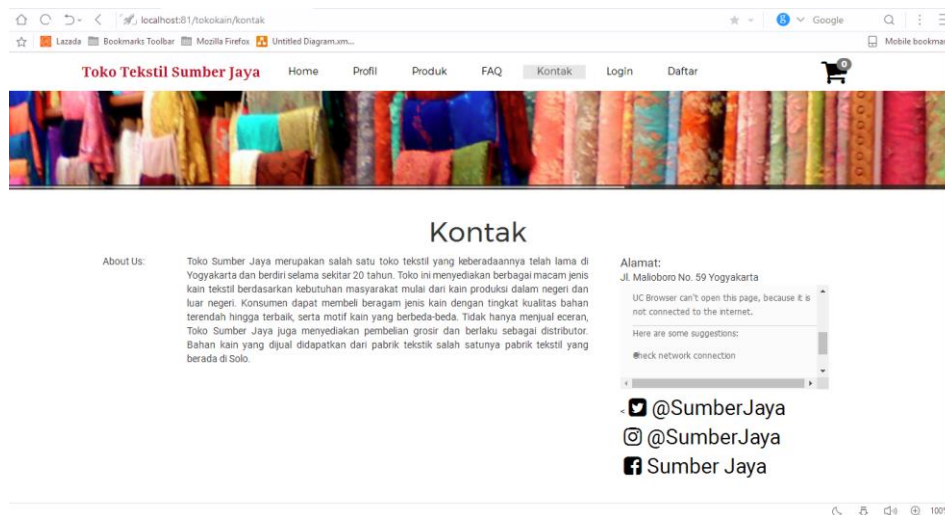
Gambar 4.22 Halaman Kontak
