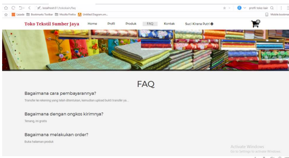
Gambar. 4.21 Halaman FaQ
