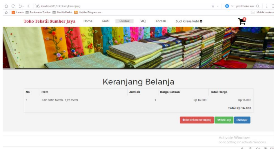
Gambar 4.15 Halaman Keranjang
