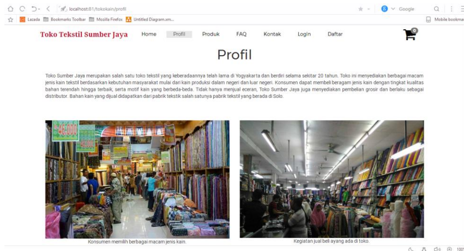
Gambar 4.12 Halaman Profil
