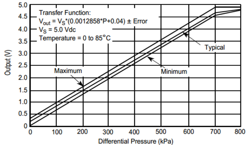
Gambar 2.2 Grafik perbandingan antara tegangan dengan tekanan[5].
