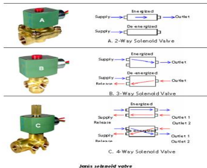
Gambar 2.5 Bentuk fisik dan simbol solenoid valve [9].
