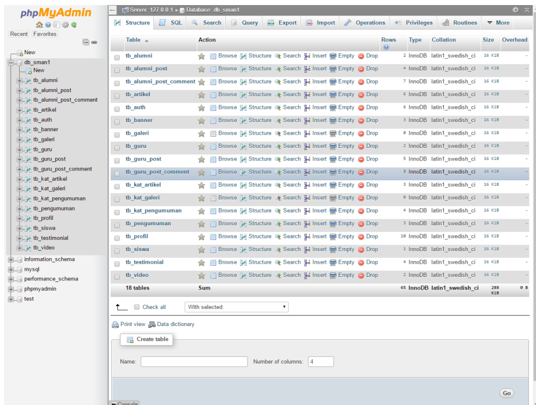
Gambar 4.2 Pembuatan Database menggunakan phpMyAdmin
