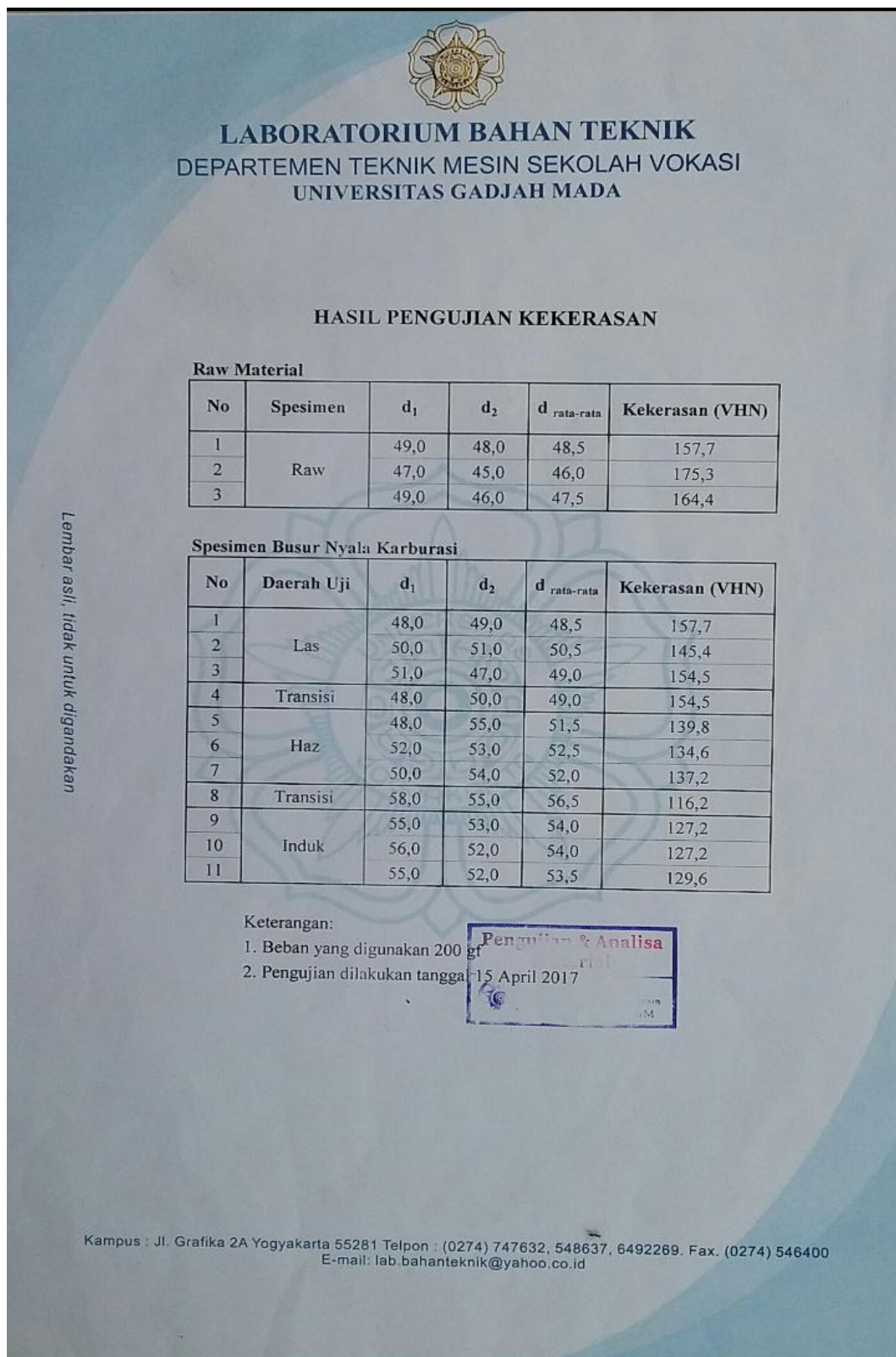
Gambar 2 Hasil pengujian Kekerasan Vickers (VHN)
