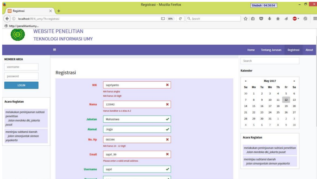
Gambar 4.7 Halaman Pendaftaran
