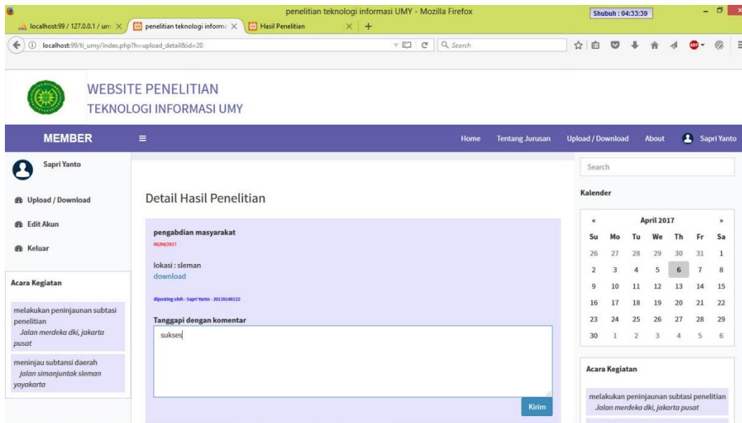
Gambar 4.14 Halaman Komentar
