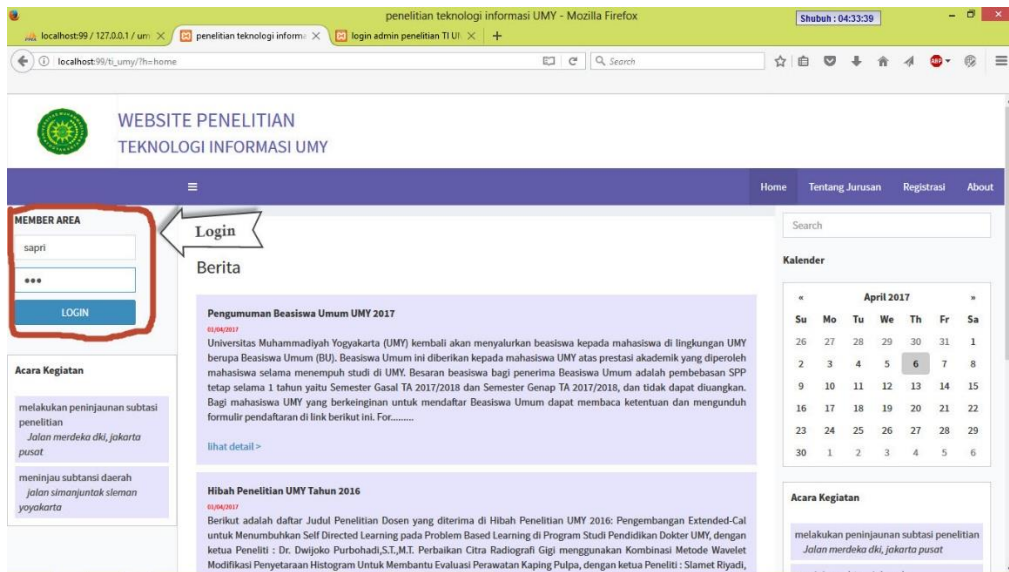
Gambar 4.9 Halaman Login
