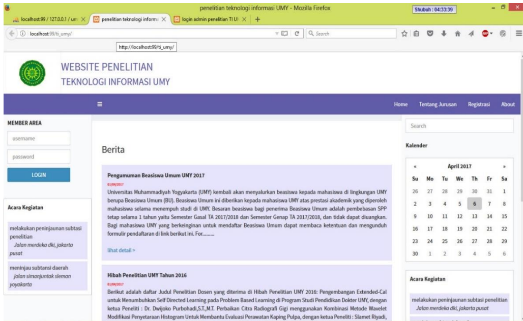
Gambar 4.8 Halaman Utama
