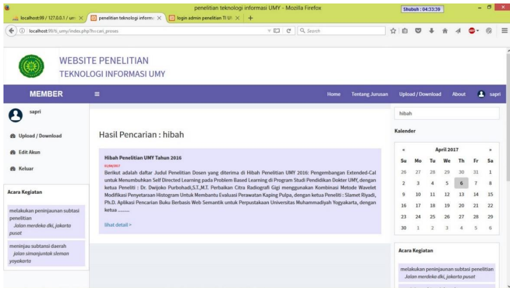
Gambar 4.13 Halaman Pencarian
